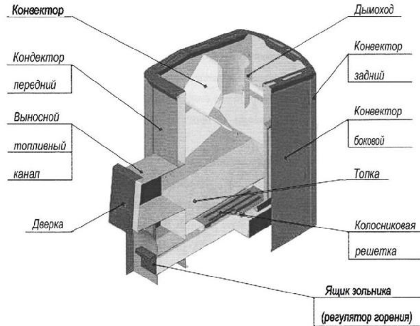
Рисунок 1 – Конструкция печи
