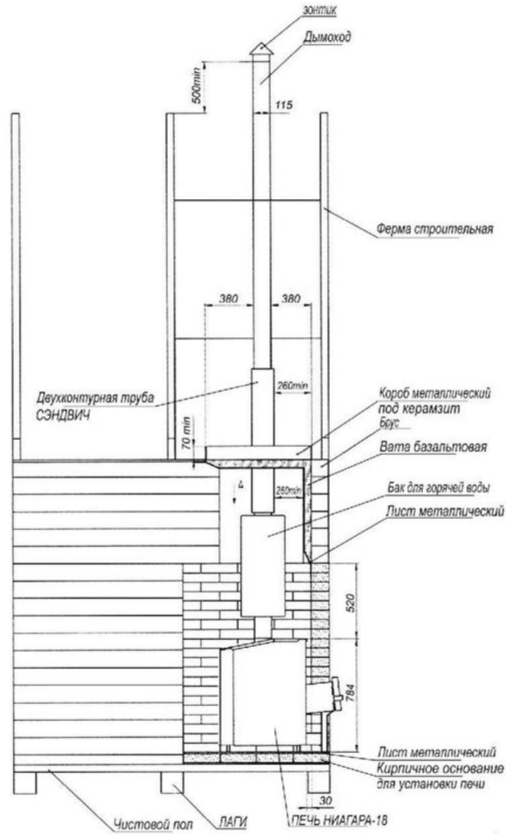
Рисунок 3 – Схема монтажа печи
