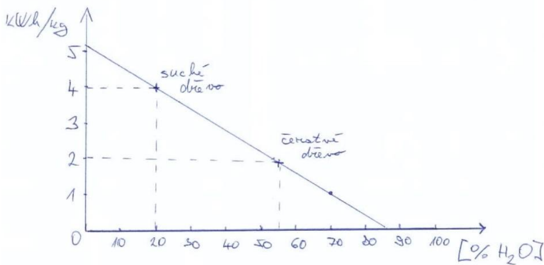
Рис. 4 График зависимости топлива и теплопроводной способности
