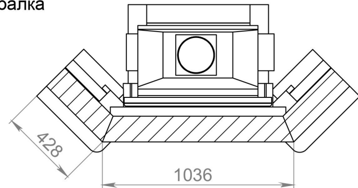
балка
